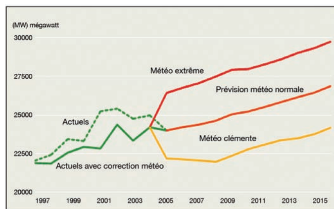
FIGURE 5 : Prévisions de la demande de pointe horaire selon trois scénarios météorologiques (Independent Electricity System Operator, 2005).
