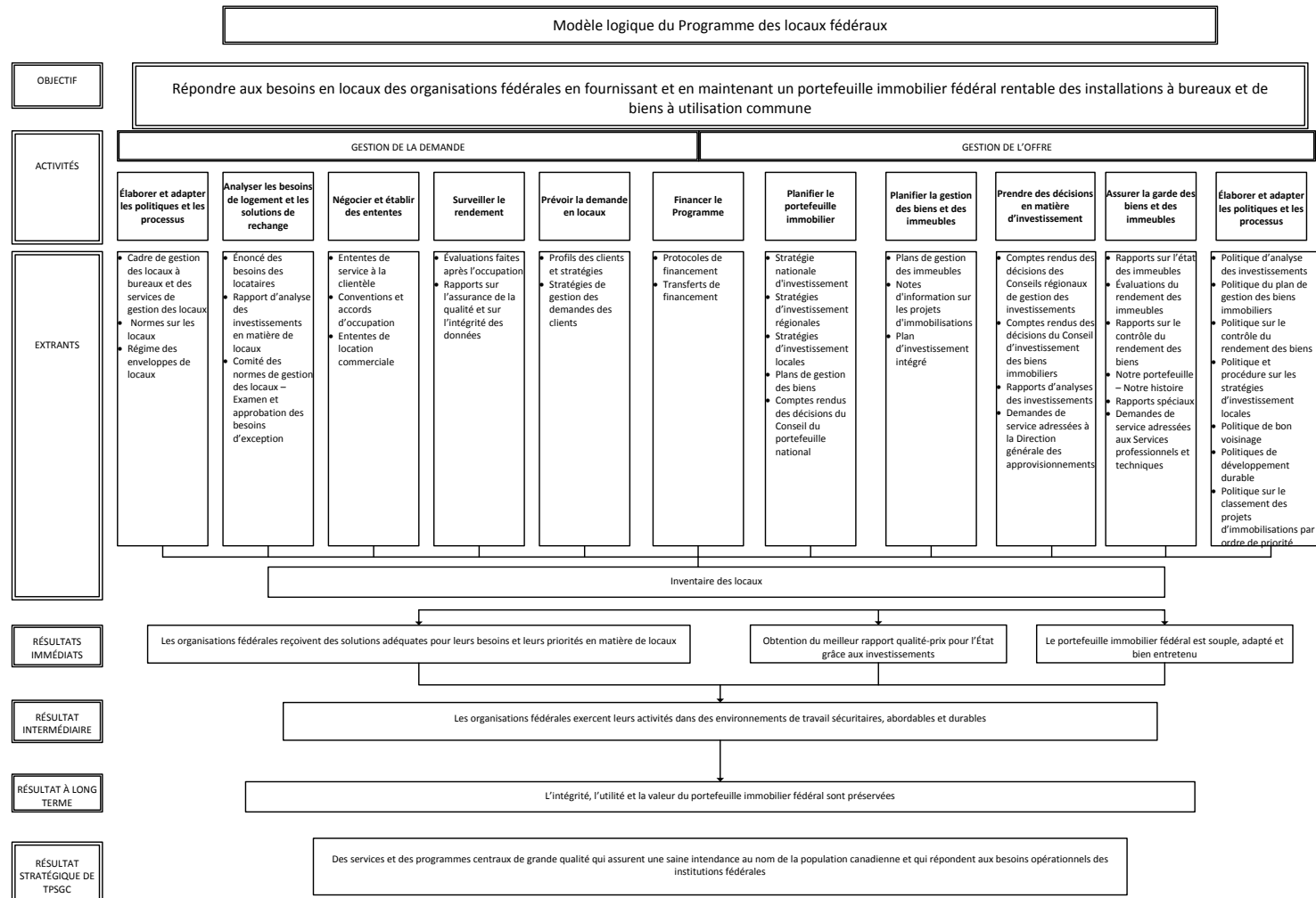
FIGURE 1 : MODÈLE LOGIQUE
